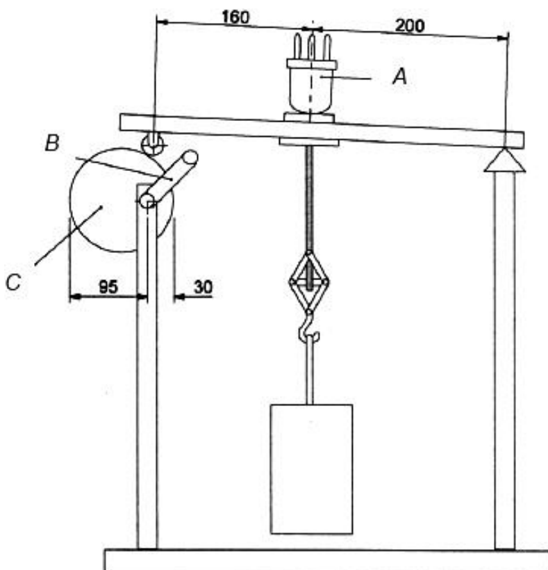
Рисунок 1 - Устройство для испытания крепления гибких кабелей натяжением
